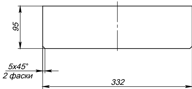
Поз.2 (Ребро) 1 : 5
